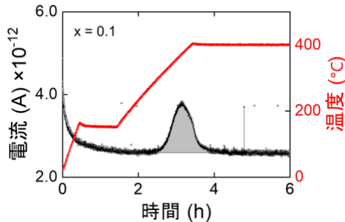
図7 TPD測定による \text{Mg}_x\text{H}_y\text{TaS}_2 からの水素放出
