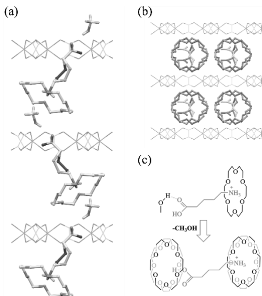
図3. 脱溶媒による結晶構造変化。(a) 2 \cdot \text{CH}_3\text{OH} の結晶構造。(b) 2 の結晶構造。(c) 脱溶媒による超分子水素結合の再配列。
