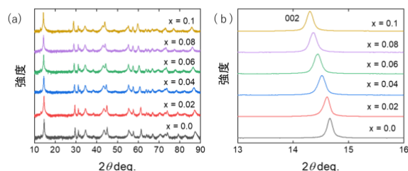
図6 (a)各Mg濃度におけるXRD測定結果 (b)002指数の拡大図
