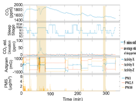
図3 閉環境 CAQLEA における各種パラメータの測定実験。上から、睡眠中の \text{CO}_2 濃度、睡眠ステージ、 \text{CO}_2 濃度の標準偏差、腕につけた加速度計の値、PM1, 2.5, 10 の各微粒子密度の時間変化を示す。
