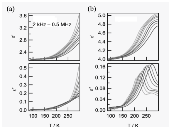
図4. 溶媒脱離前後の誘電率の温度周波数依存性。(a) 結晶 2 \cdot \text{CH}_3\text{OH} 。(b) 結晶 2 。
