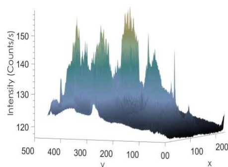
図 10. 平均化された Raman 画像を波数軸に沿って示した強度分布
