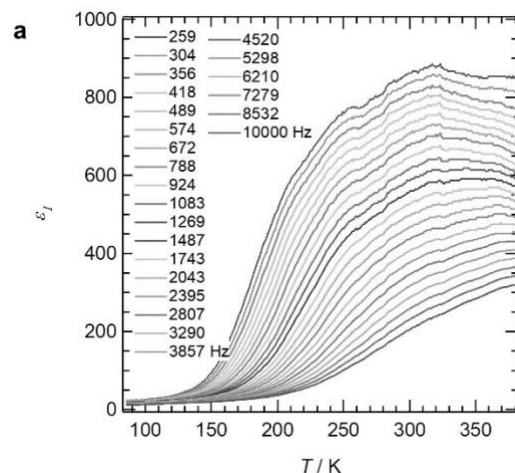
図2. 複素誘電率実部の温度周波数依存性。測定周波数が高周波数であるほど、複素誘電率実部のピークが高温側にシフトしている。
