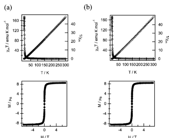
図5. 溶媒脱離前後の磁化率の温度依存性(上)と磁場依存性(下)。(a) 結晶 2 \cdot \text{CH}_3\text{OH} 。(b) 結晶 2 。
