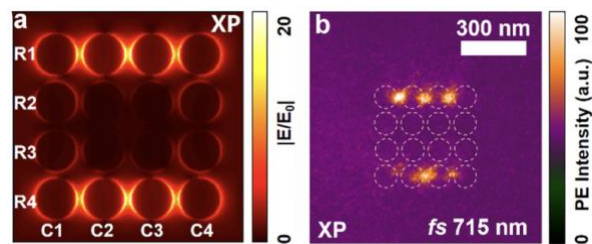
図2 正方格子のエッジ状態 (a)シミュレーション、(b)PEEMによる近接場イメージ。
