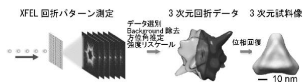
図2 MAXIC-Sを用いた溶液中金ナノトライアングルの3次元イメージング
